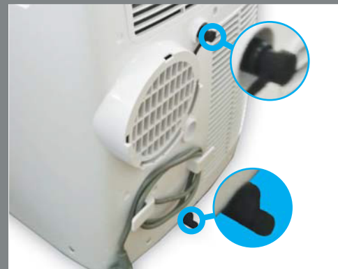
Doppelter Kondensatablauf
